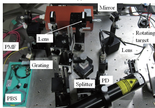
図 2. 実験系 構成図と実験装置写真
