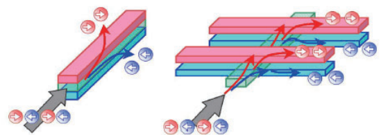
図6. 電流を流すだけでスピン流を発生させるスピン・ホール効果の例 (左) 電流が流れている間のみスピン流が発生 (右) 異方性の付与により電流で磁性を制御
