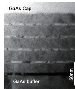
図3. 作製した異種磁性層のナノ周期積層構造
