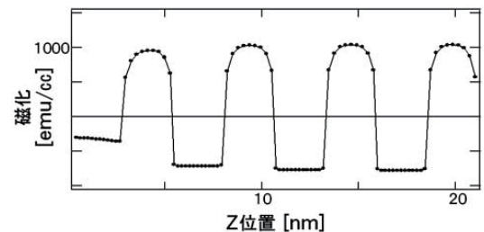
図5. 理論シミュレーションによる積層磁性体内部のスピン状態
