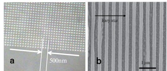
図4. 半導体上に設計製作された面内パタニングによる周期アレイ・ストラクチャー (a) ドット (b) ライン
