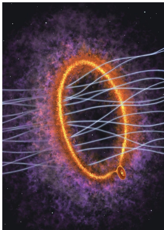
図1: アルマ望遠鏡の観測に基づく分子雲コア MC 27 内部の想像図。 右下にあるのが原始星およびその周りを取り巻く円盤であり、そこからリング状に暖かいガスが広がっている。リングの内部には磁力線が貫いている。 (Credit: Y. Nakamura, K. Tokuda et al.)
