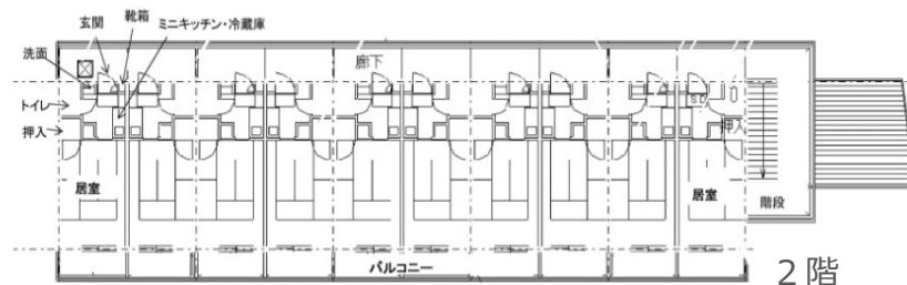
平面図
