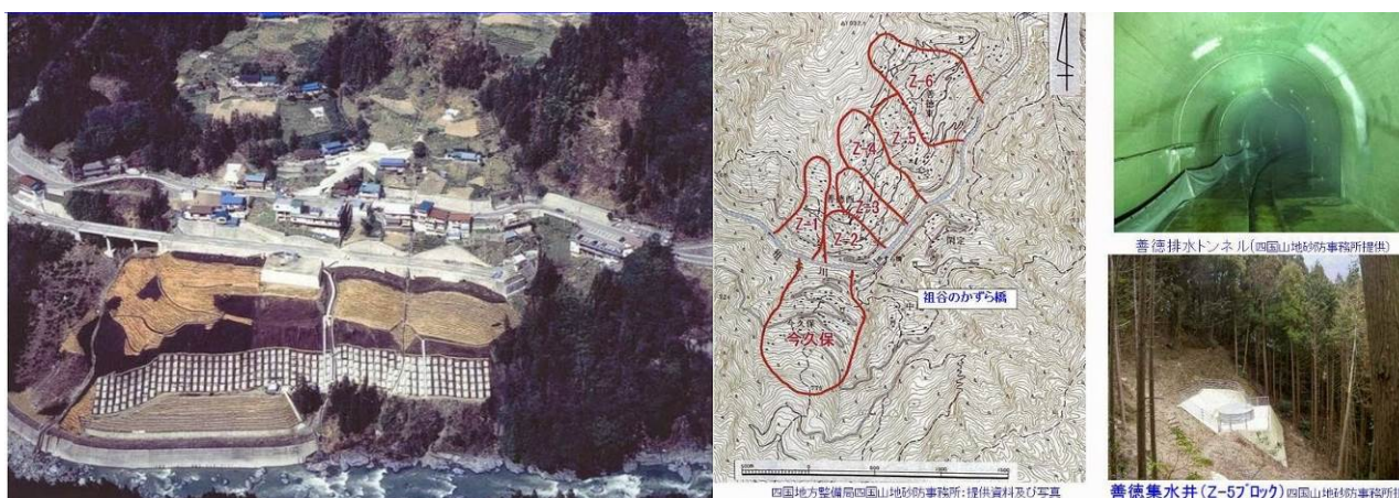
写真2 今久保地区の地すべり対策の全景 (2007年撮影)
