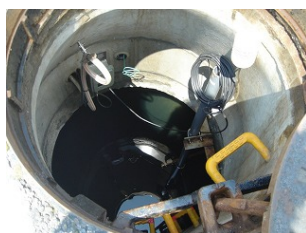
排水枡 pH計センサー
