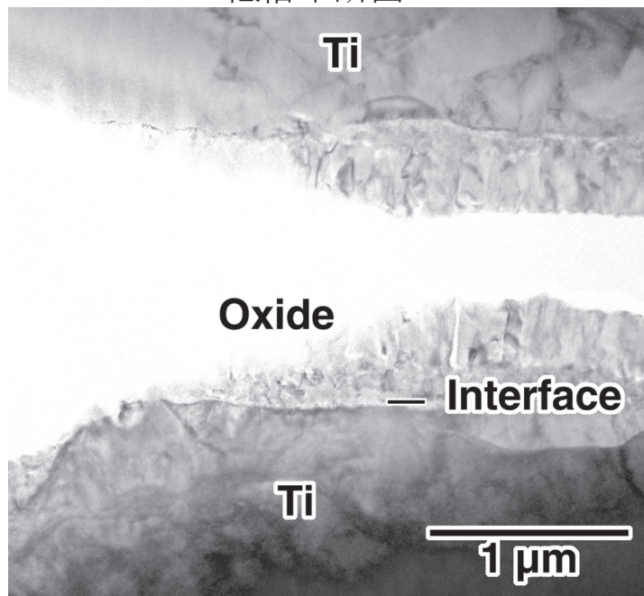
低倍率断面
