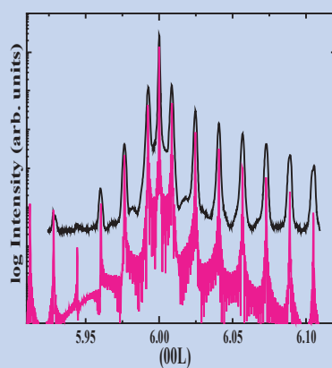
X線超格子反射測定
