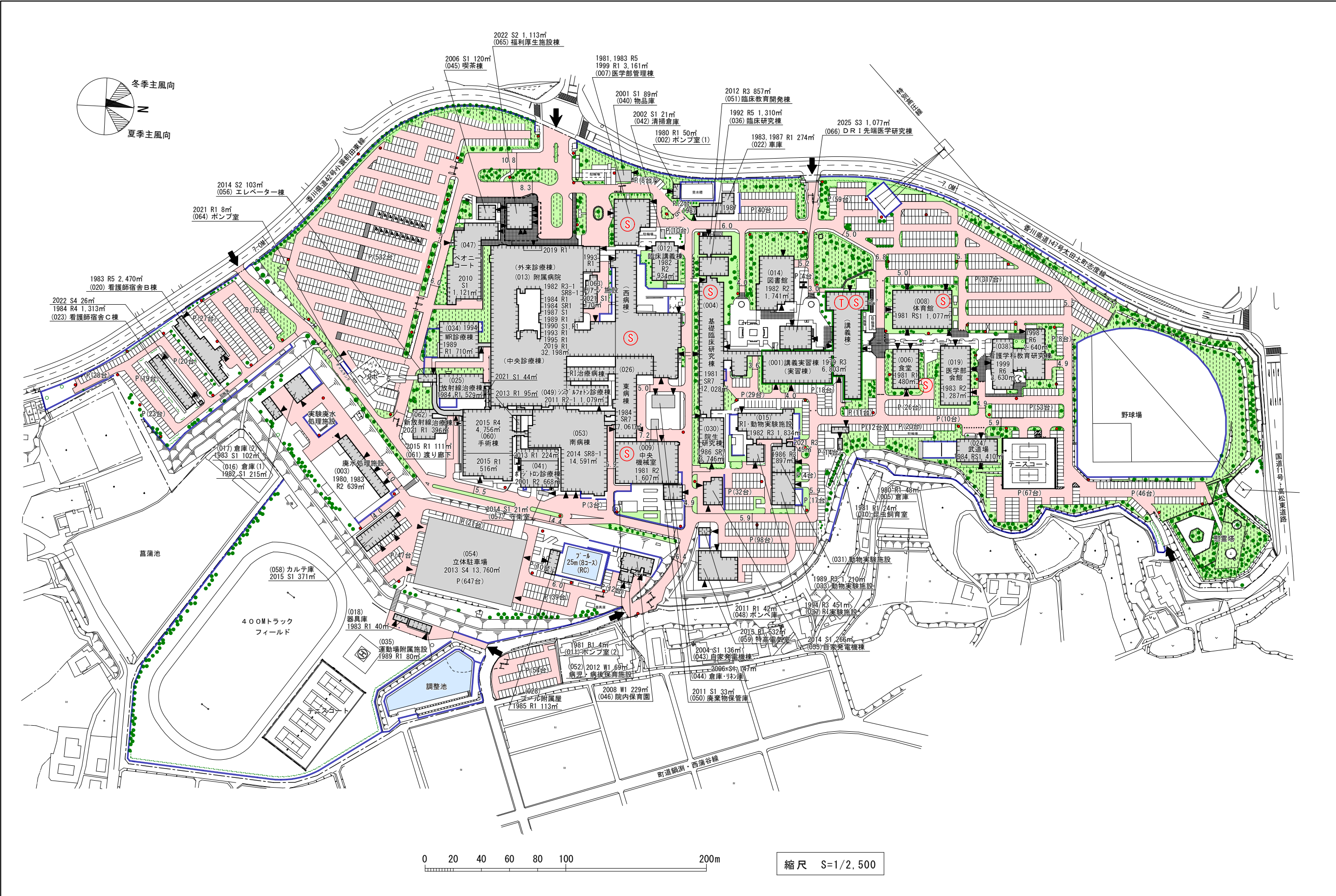
(3) 校舎・運動場等の配置図
