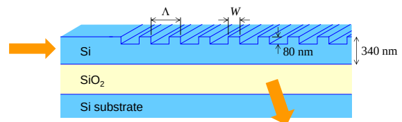
図2 グレーティングカプラのモデル
