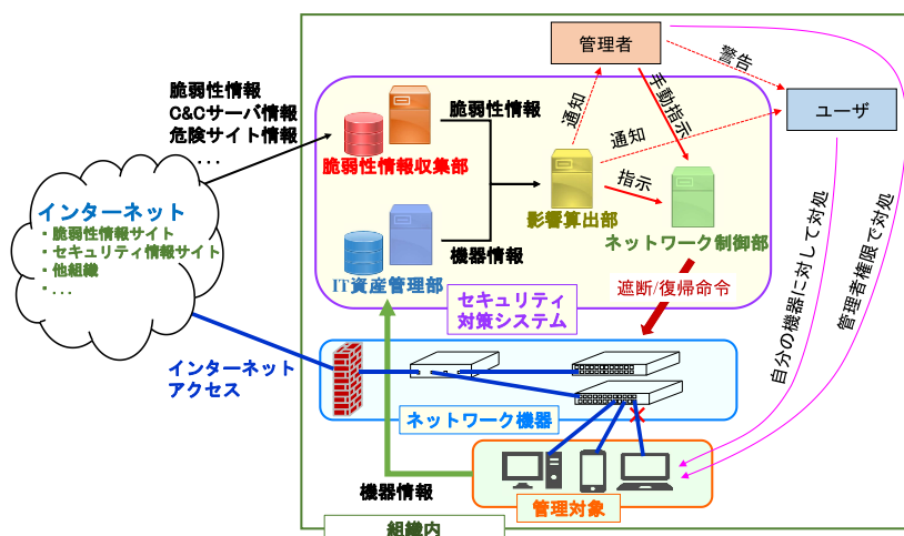
図1 情報セキュリティ対策システムの概要
