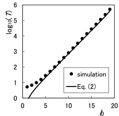
図2 過渡回転波の持続時間 T vs 初期パルス幅 l_0
