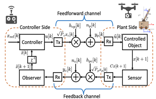
図2 無線制御システム
