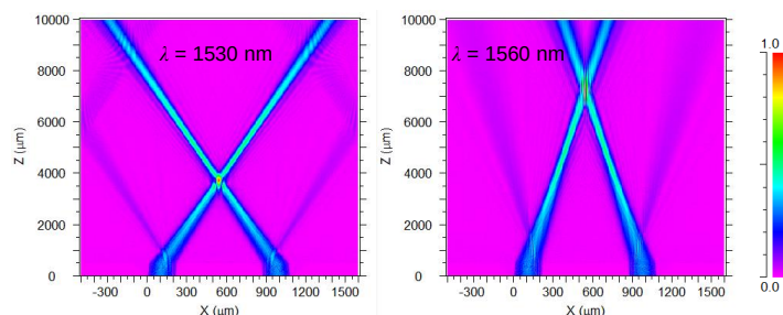
図3 出射光電界振幅分布の計算例
