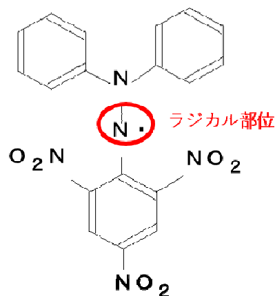
DPPHラジカルの化学構造
