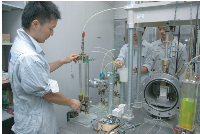
写真 1 透水試験風景
